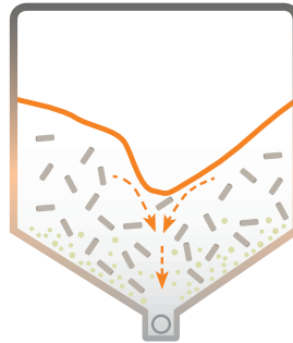
Sanduhreffekt bei der Entnahme von Pellets
